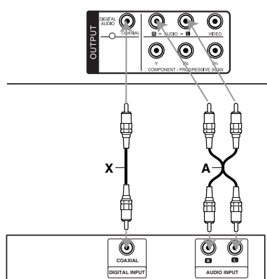
Amplificador (Receptor)
