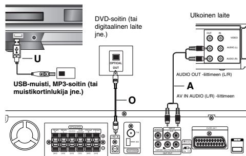
DVD/CD-vastaanotin takaa
