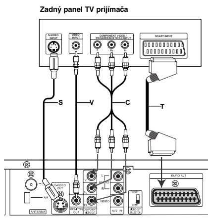
Zadný panel DVD/CD prehrávača
