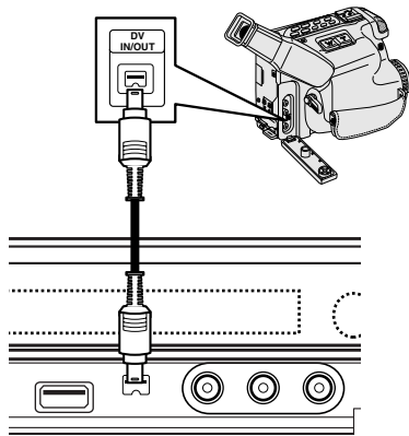
Panel delantero de la grabadora
