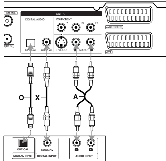
Amplificateur (Récepteur)
