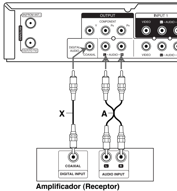
Panel posterior del grabador
