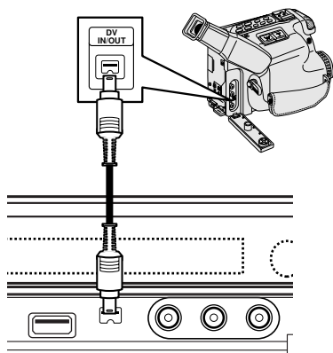
Přední strana rekordéru
