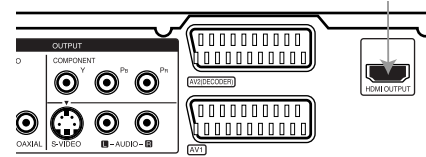
Zadní část rekordéru
