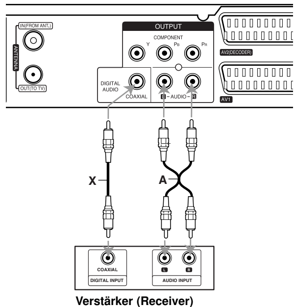
Rückseite des Rekorders
