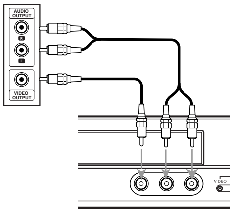
Vorderseite des Rekorders
