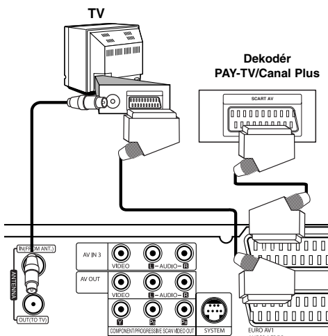
Zadná strana HDD/DVD rekordéra
