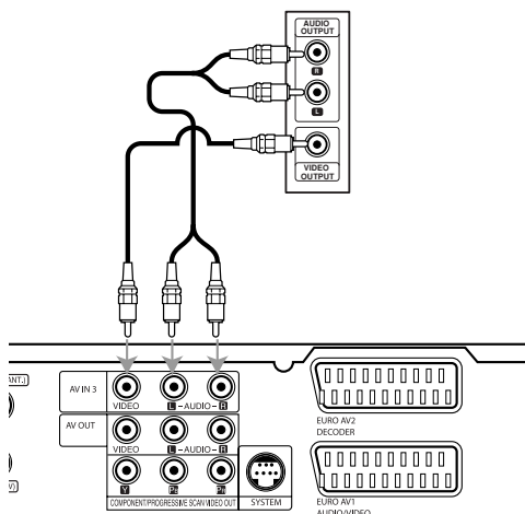
Zadná strana HDD/DVD rekordéra
