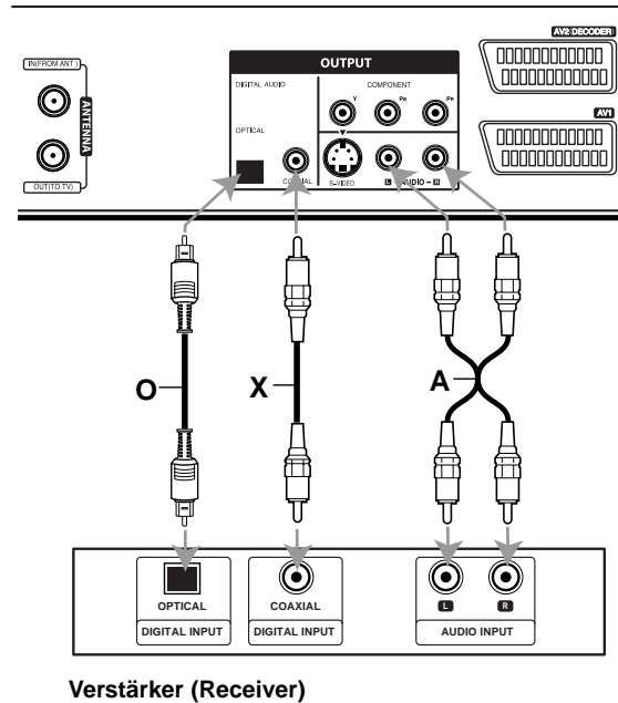
Verstärker (Receiver)
