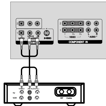
Cable Box
