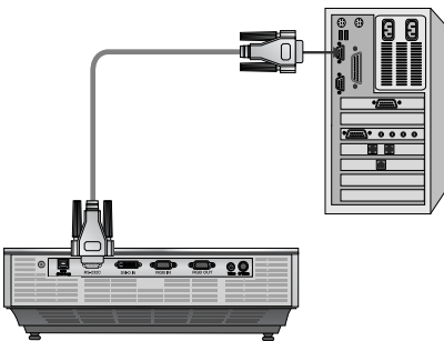
<Fig. 1, câble d'interface RS-232>
