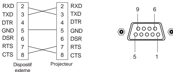
<Fig. 1, câble d'interface RS-232>
