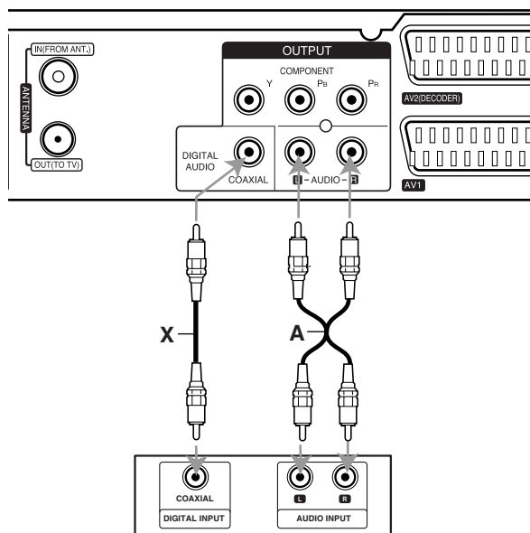
Amplificateur (Récepteur)
