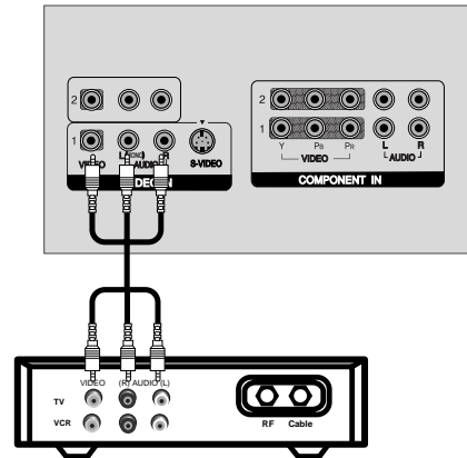
有线机顶盒
