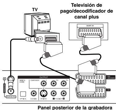
Panel posterior de la grabadora
