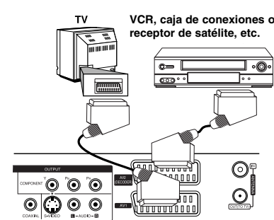
Panel posterior de la grabadora
