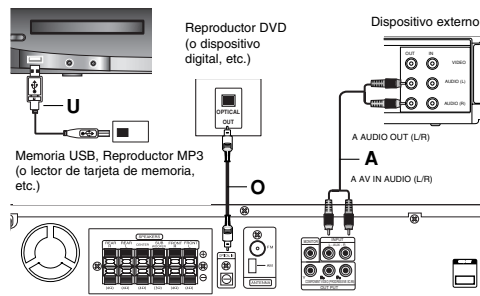
Parte trasera del receptor de DVD/CD
