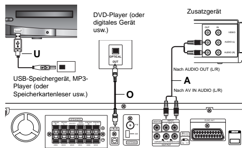
Rückseite des DVD/CD-Receivers
