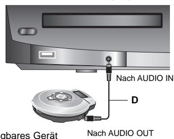
Tragbares Gerät Nach AUDIO OUT
