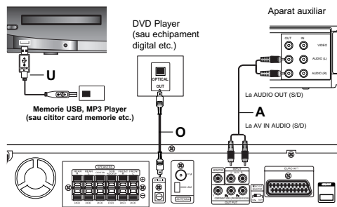
Partea din spate a DVD/CD Receiver-ului
