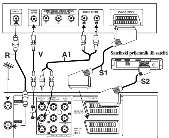
Zadnji panel ovog aparata (osnovni spojevi)
