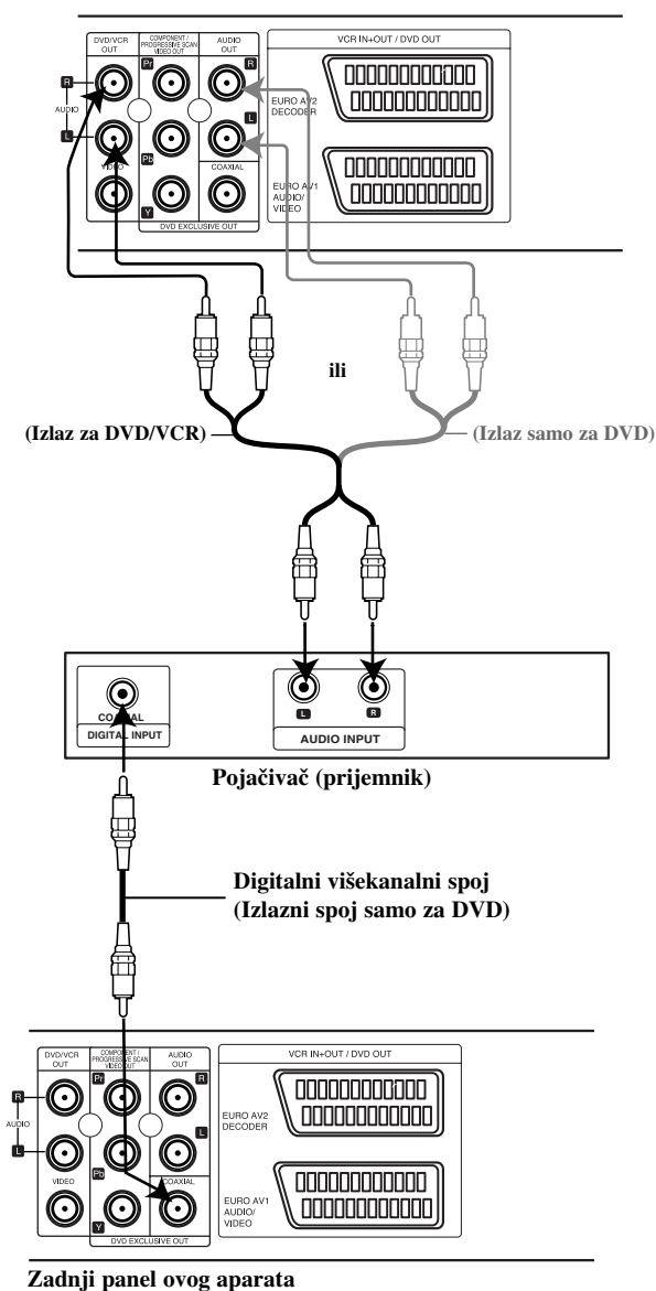
Zadnji panel ovog aparata
