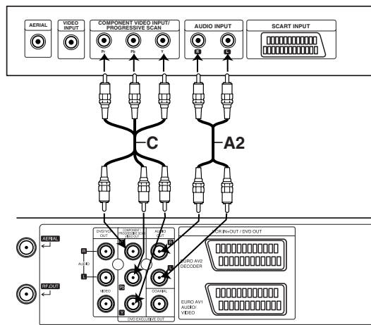
Zadnji panel ovog aparata (osnovni spojevi)
