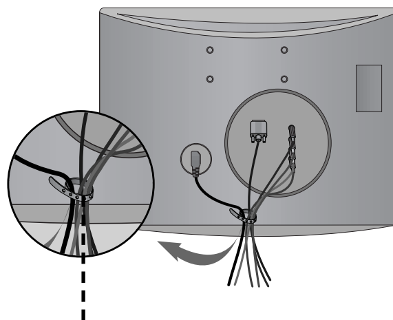
Upevňovač káblov
