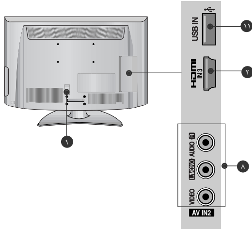
(بالنسبة للطرز (32/37/42/47LH3***
