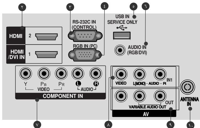
(بالنسبة للطرز (26/32/37/42LH2***
