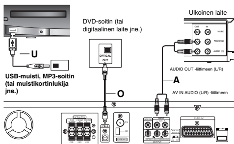
DVD/CD-vastaanotin takaa
