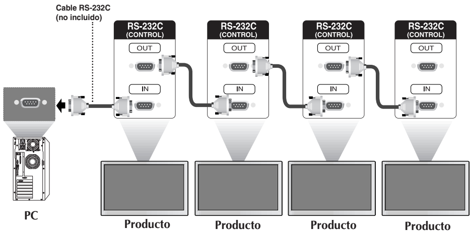
Configuraciones para cable de 7 hilos (cable RS-232C estándar)
