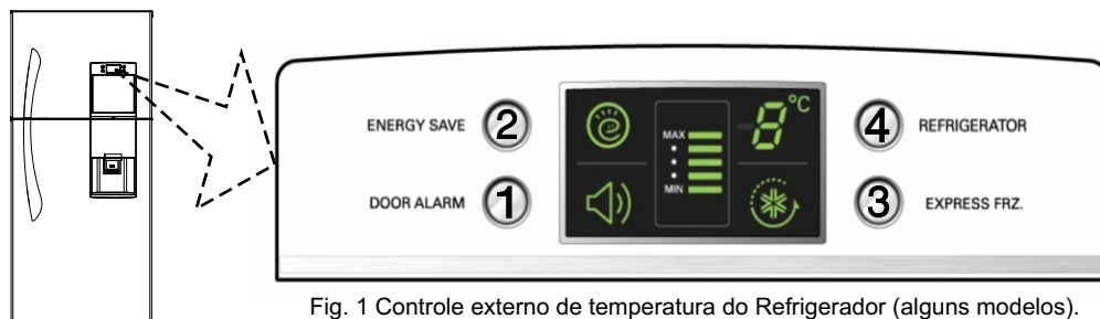
Fig. 1 Controle externo de temperatura do Refrigerador (alguns modelos).
