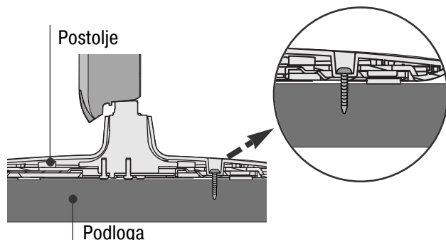
1-vijak (dostavljen kao dio proizvoda)
