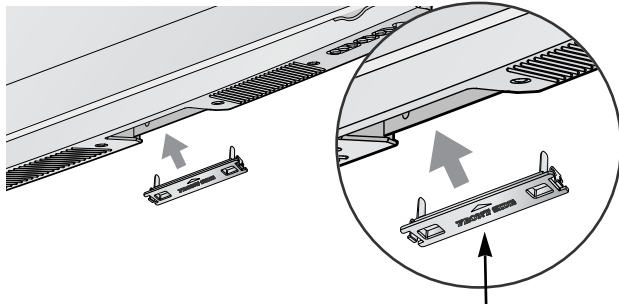
Capac protecție
