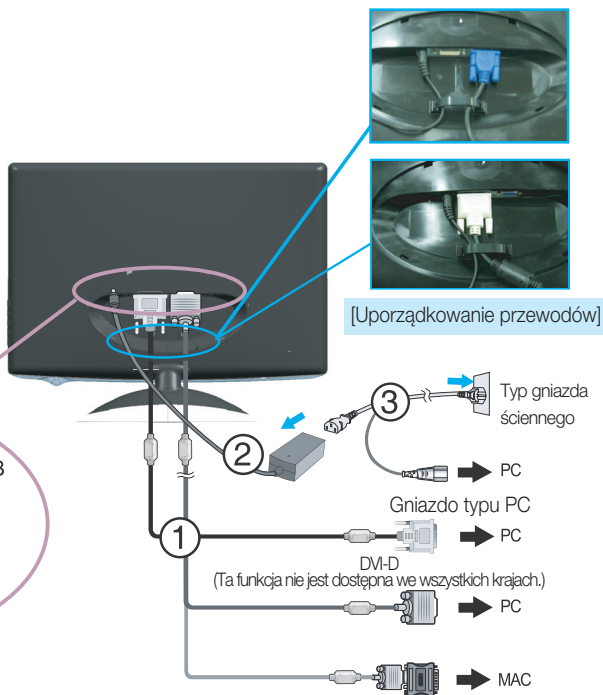
[Podłączanie przewodów]
