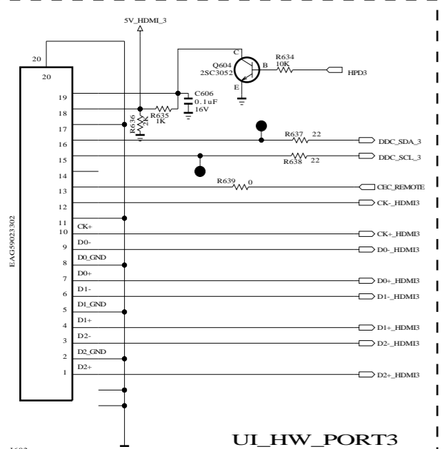
UL_HW_PORT3
