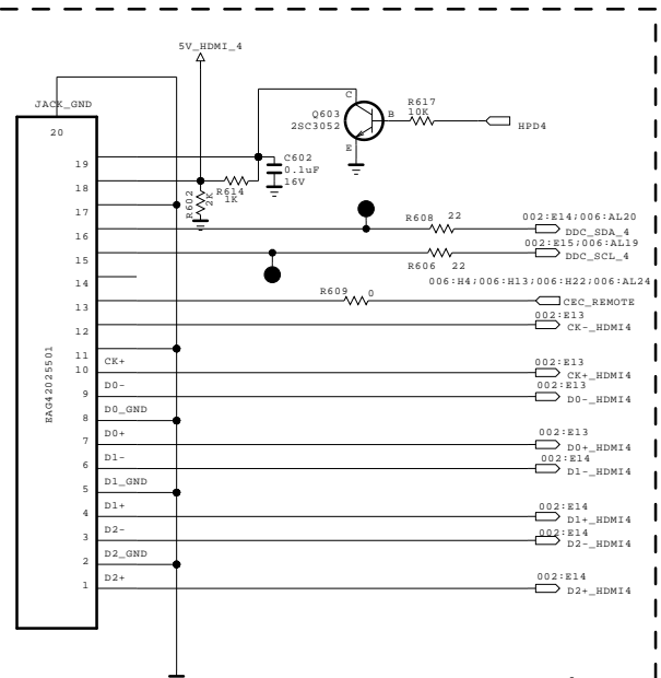
UI_HW_PORT4
