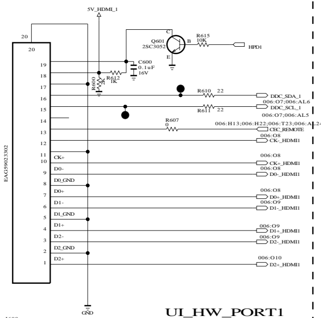
UL_HW_PORT1
