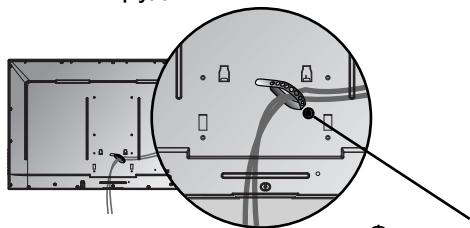
Фиксатор проводов
