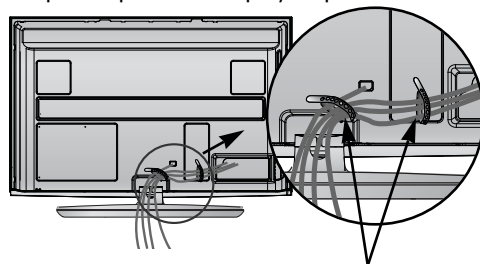
Στήριγμα Καλωδίου
