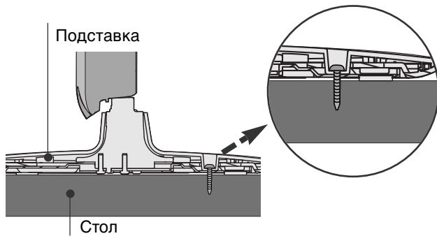
Подставка
