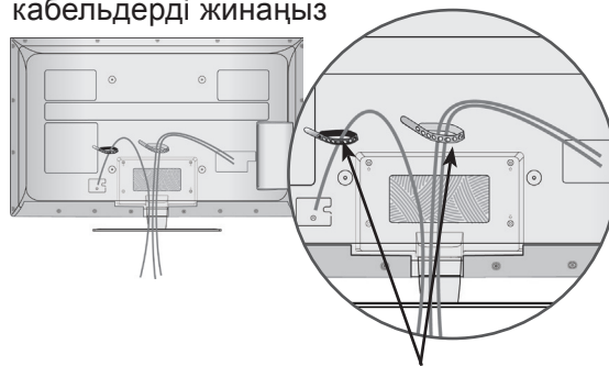
Кабель ұстатқыш
