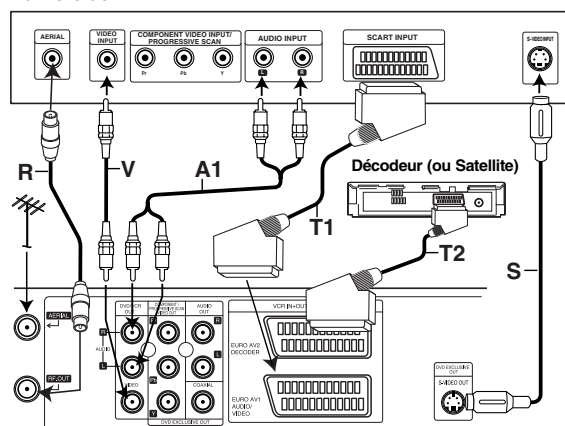
L'arrière de l'appareil (Branchement de base)
