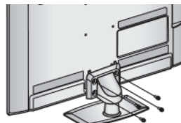
M4 X 14 (Pouze 26LE3***, 26LE5***)
