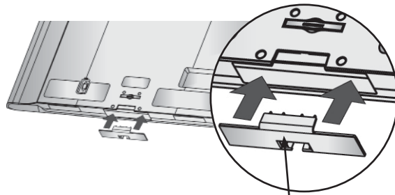
Предпазен капак
