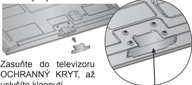
Ochranný kryt
