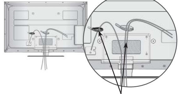
ΣΤΗΡΙΓΜΑ ΚΑΛΩΔΙΟΥ
