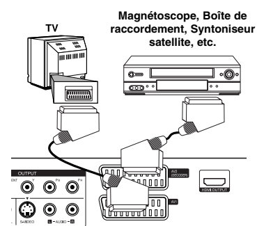
Panneau arrière du graveur
