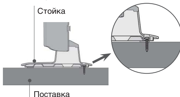
Поставка
