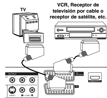
Panel posterior de la grabadora
