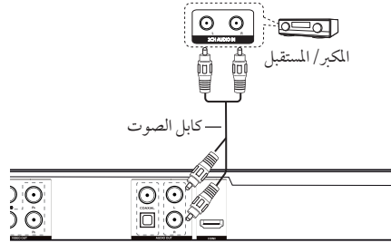
الجزء الخلفي من الوحدة
