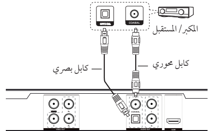
الجزء الخلفي من الوحدة
