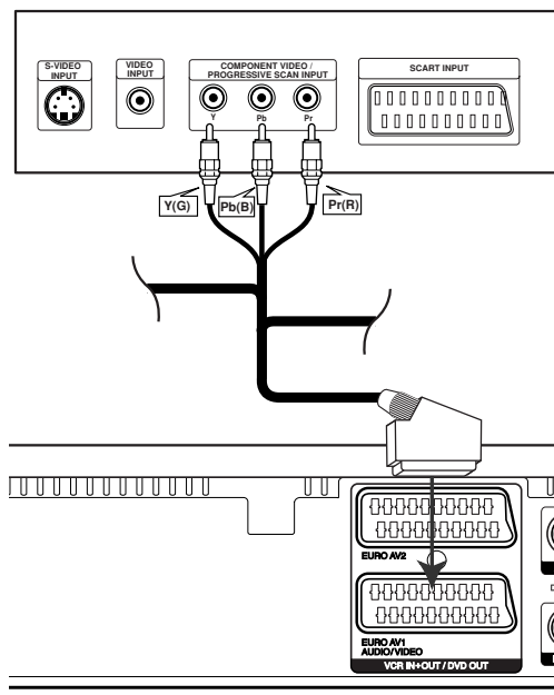
Stražnji panel KOMBINIRANI DVD/VCR
