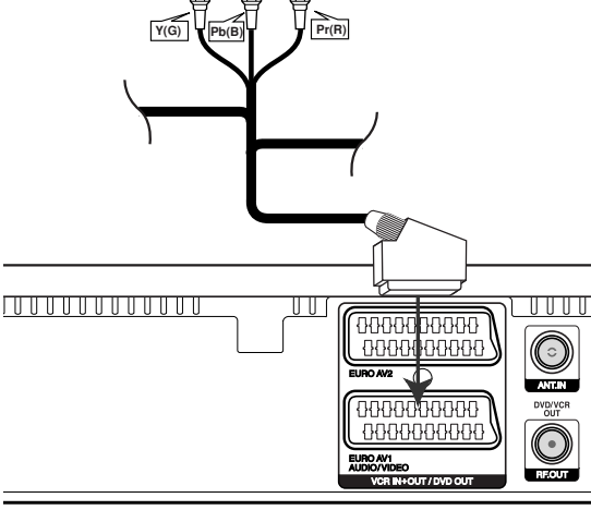
Zadní část KOMBINOVANÝ PŘÍJÍMAČ DVD/VCR
