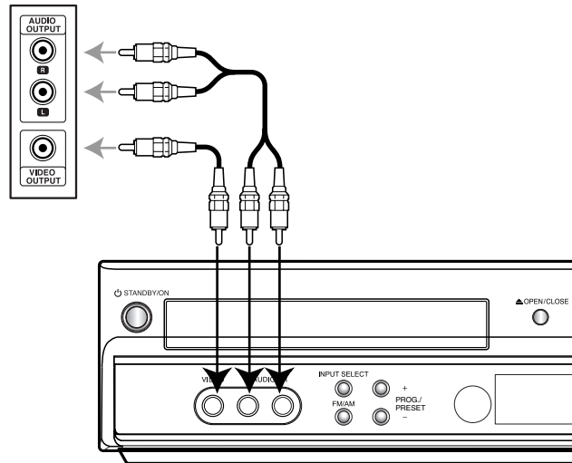
Panel konektorů přídavného zařízení
