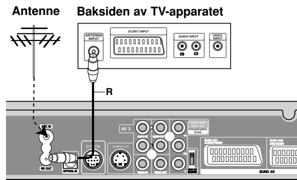
Baksiden av HDD/DVD-opptaker/mottakeren
