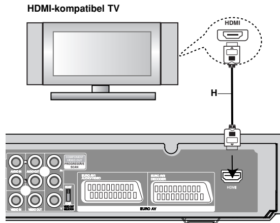
Baksiden av HDD/DVD-opptaker/mottakeren
