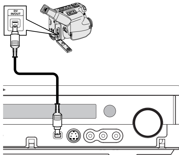
Fronten på HDD/DVD-opptaker/mottakeren
