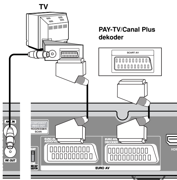
Baksiden av HDD/DVD-opptaker/mottakeren
