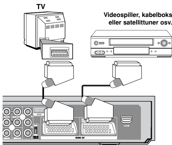
Baksiden av HDD/DVD-opptaker/mottakeren
