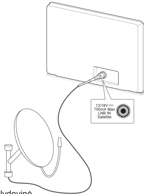
Palydovinė antena
