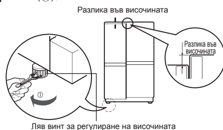
Ляв винт за регулиране на височината
