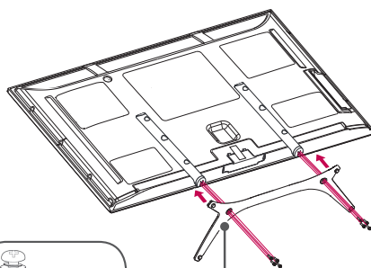
Základňa stojana
