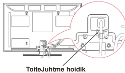
Toitejuhtme hoidik
