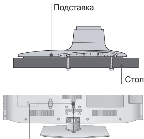
1 – Винт (поставляется вместе с изделием)
